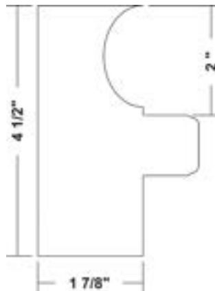
CAR-BN-RC-APC
