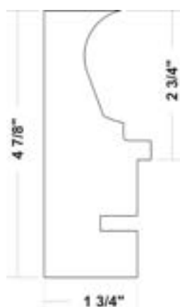
CAR-CRC-FGWT
